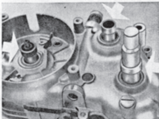
Buchse für Simmerringschutz Ersatzteil 15 \varnothing = 09.30.34 - 2/351 17 \varnothing = 09.30.11 - 2/344 20 \varnothing = 09.30.35 - 2/352
